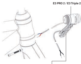
Multimount CS (Enthalten im Lieferumfang des E3 PRO 2 / E3 Triple 2) (Included at V1260 / E3 PRO 2 / E3 Triple 2) (Compris dans le contenu des phares E3 PRO 2 / E3 Triple 2) (inbegrepen bij de levering van de E3 PRO 2 / E3 Triple 2)
