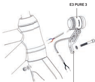
Multimount HSOP (Enthalten im Lieferumfang des E3 PURE 3) (Included at V521s / E3 PURE3) (Compris dans le contenu des phares E3 PURE 3) (inbegrepen bij de levering van de E3 PURE3)
