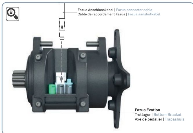
Anschlusskabel Kopplung | Connecting to drive cable Câble de raccordement pour le branchement | Connectie van de aansluitkabel
