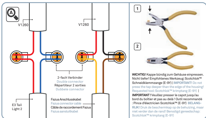
V1260 & E3 Tail Light 2 (6 V) Verbindung zum Fazua Anschlusskabel | V1260 & E3 Tail Light 2 (6 V) connection to Fazua connection cable Connexion du V1260 & E3 Tail Light 2 (6 V) au câble de raccordement Fazua V1260 & E3 Tail Light 2 (6 V) Connectie van de Fazua aansluitkabel
